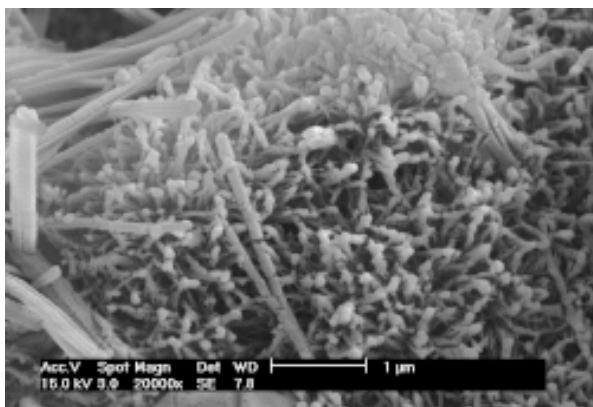
Microfoto van de cementmatrix van met water aangemaakte Keracolor
