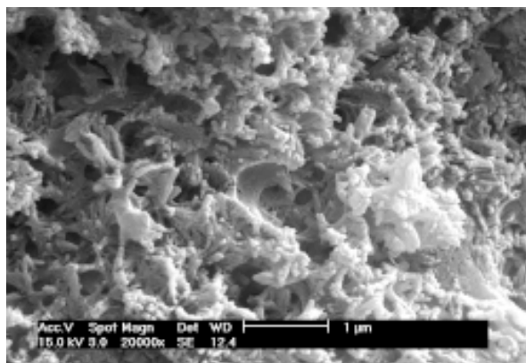
Microfoto van de cementmatrix van met Fugolastic aangemaakte Keracolor . Let op de veel compactere structuur door de in de tussenruimten aanwezige polymeren
